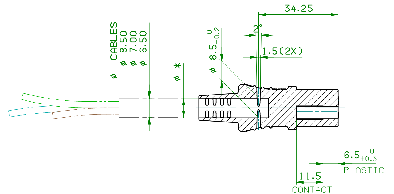
SECCIÓN A-A
